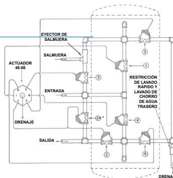
Actuador (Modelo 48-00)
